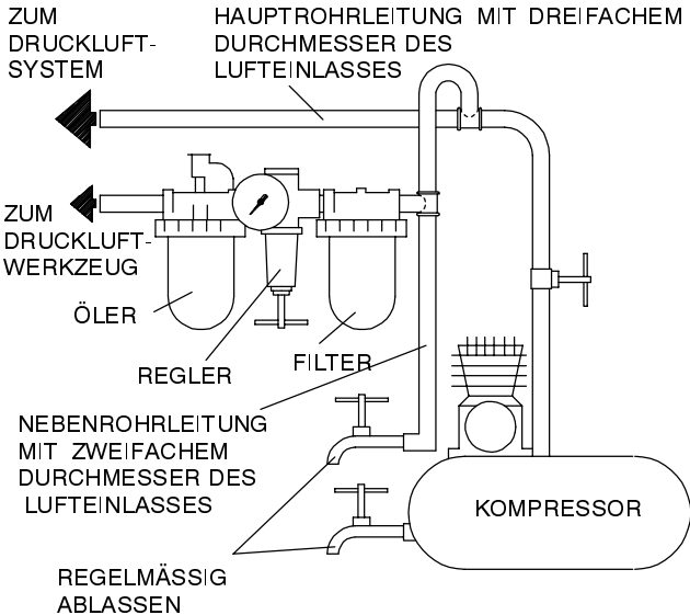
(Zeichn. TPD905-1)
